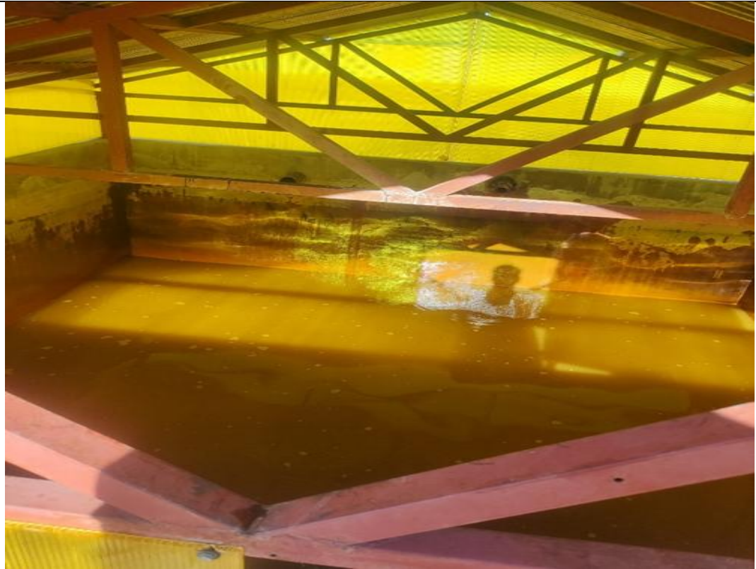
Reservorio de agua cruda y línea de conducción – Imagen del reservorio con acumulación de sedimentos, sujeto a limpieza y desinfección mensual según normativa DIGESA. Y vista de la tubería de entrada de agua cruda antes del tratamiento de la PTAP
